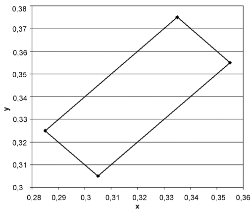
Rys. 1. Współrzędne chromatyczności x,y dla barwy białej oznakowania
