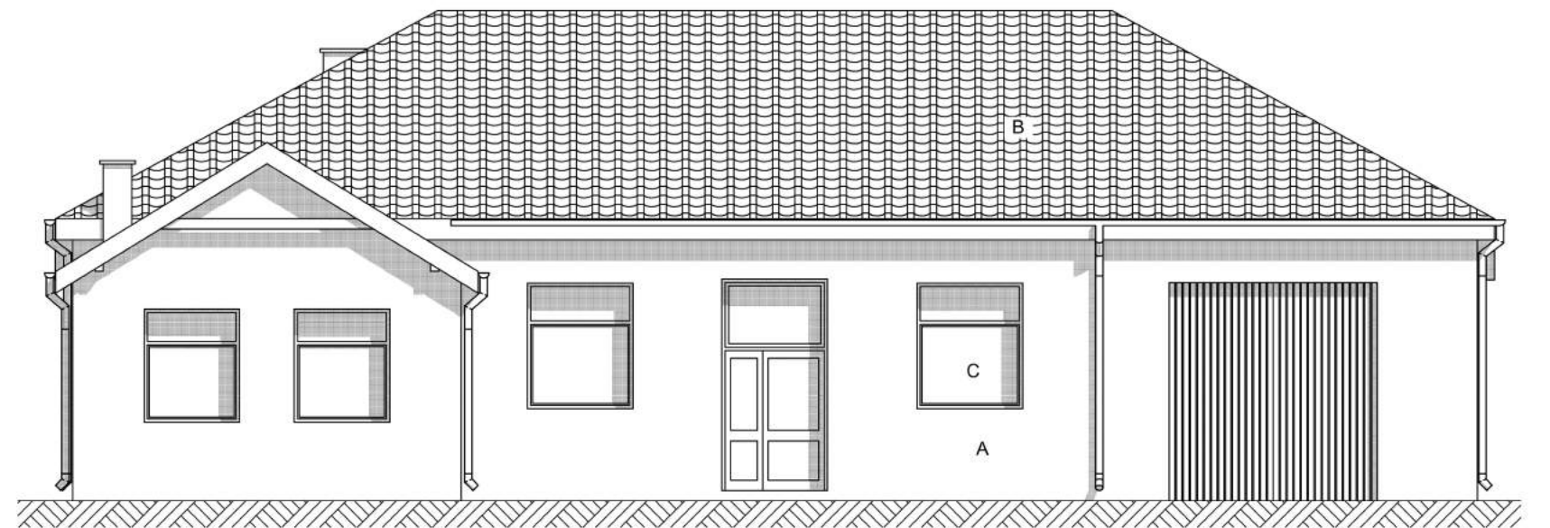
Elewacja Południowa
