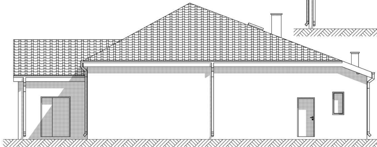
Elewacja Wschodnia
